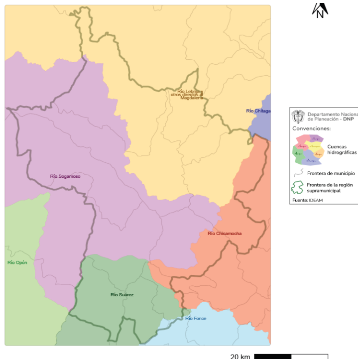
Gráfico 45 Cuencas hidrográficas de la región supramunicipal, nodo Bucaramanga Fuente: (Sistema de Planeación Territorial, 2023)
